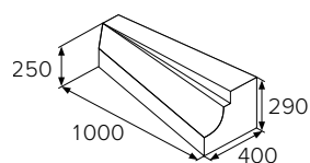
BEST ZASTÁVKOVÝ OBRUBNÍK přechodový 250/290
