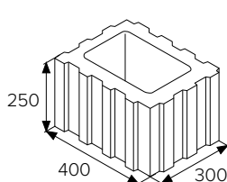
BEST KASKADA II
