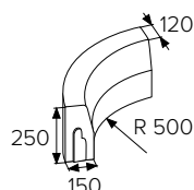
BEST MONO II R0,5 vnitřní
