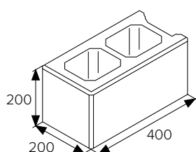
BEST LUNETA IV (koncový prvek)
