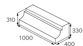
BEST ZASTÁVKOVÝ OBRUBNÍK náběhový 310/330
