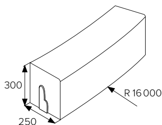
BEST KERBO R16 vnější
