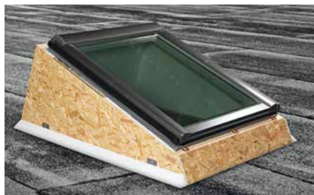
Sklon okna ve zdvihovém rámu je zvýšen o bezpečných 20° proti zatékání
