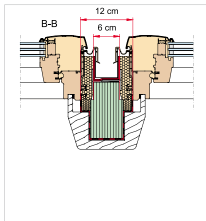
Kombinace pomocné krovky EKS s obložením z masivního dřeva v bílé barvě pro jiný systém ostění než Roto ZIN
