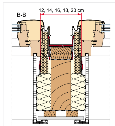
Standardní kombinace bez pomocné krovky EKS
