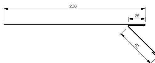
FSRP Zatahovací okapový plech, r. š. 307,5 mm
