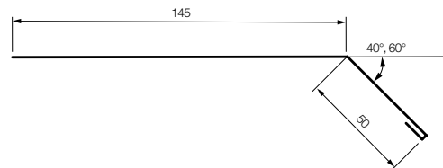
FOTPA – okapový plech, r. š. 245 mm
