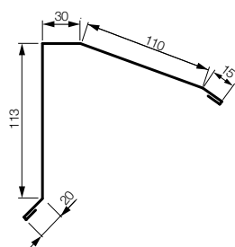
VISK-S – závětrná lišta pro taškovou krytinu – spodní, r. š. 307,5 mm
