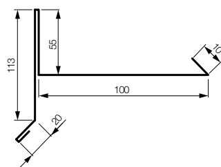
VISK-S – závětrná lišta pro taškovou krytinu – spodní, r. š. 307,5 mm
