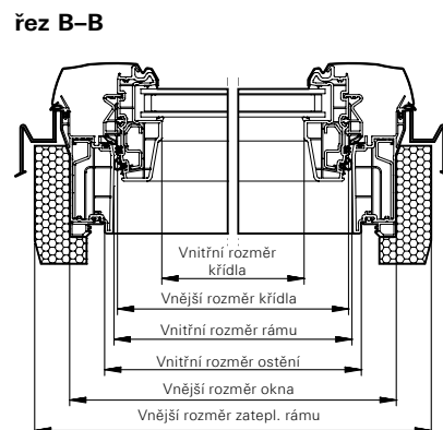
řez B-B
